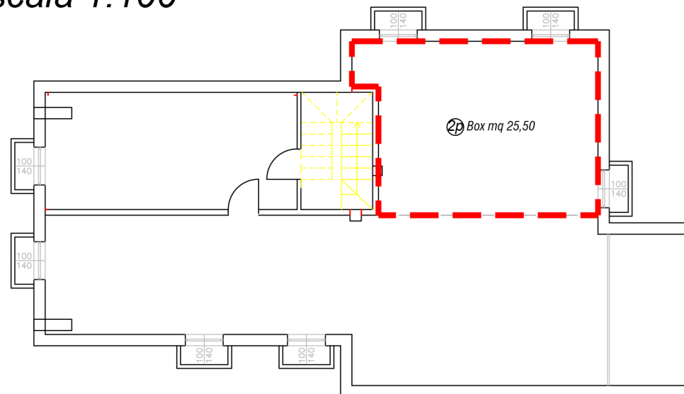
Piano interrato - scala 1:100
