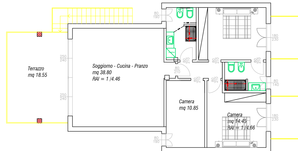
Piano Primo - APPARTAMENTO N° 2p ARREDATA scala 1:100
